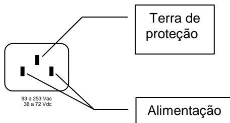
Figura 2. Conector da fonte de alimentação
